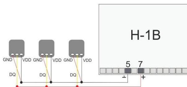
Датчик DS18B20
